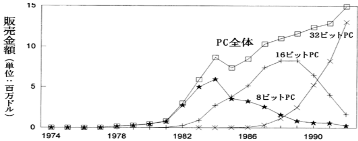
図4 CPU のビット数別販売金額の歴史的推移(1974-1992)
