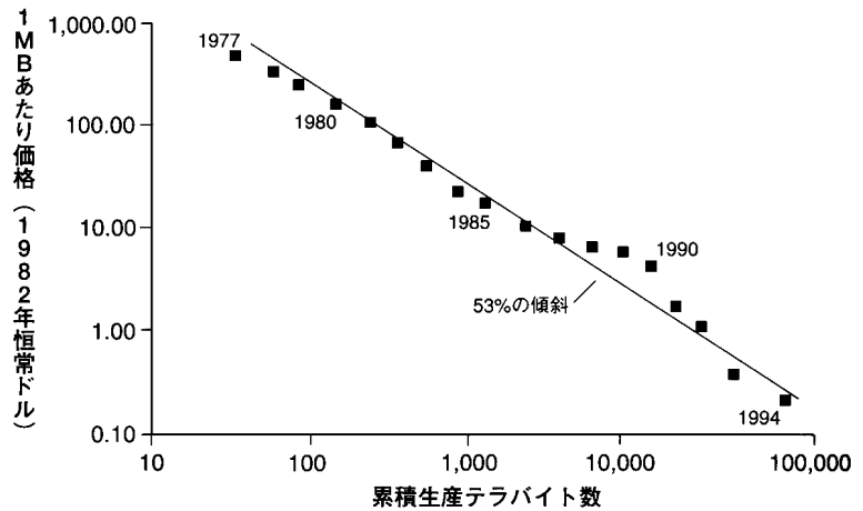
図1.3 ディスク・ドライブ価格の経験曲線 資料: 「ディスク/トレンド・レポート」各号のデータ
