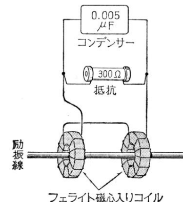
図15 パラメロン素子
