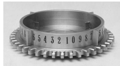
図8 階差機関の歯車
