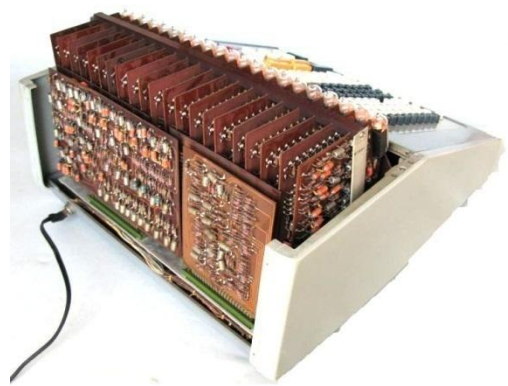
図14 コンペット CS-10A の内部の写真
