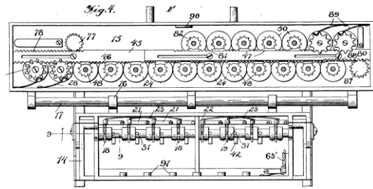
図4 ボールドウインの特許申請図(1889)
