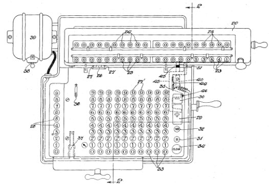
図11 モンロー社の電動電卓
