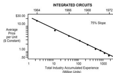
図2 半導体集積回路に関する経験曲線
